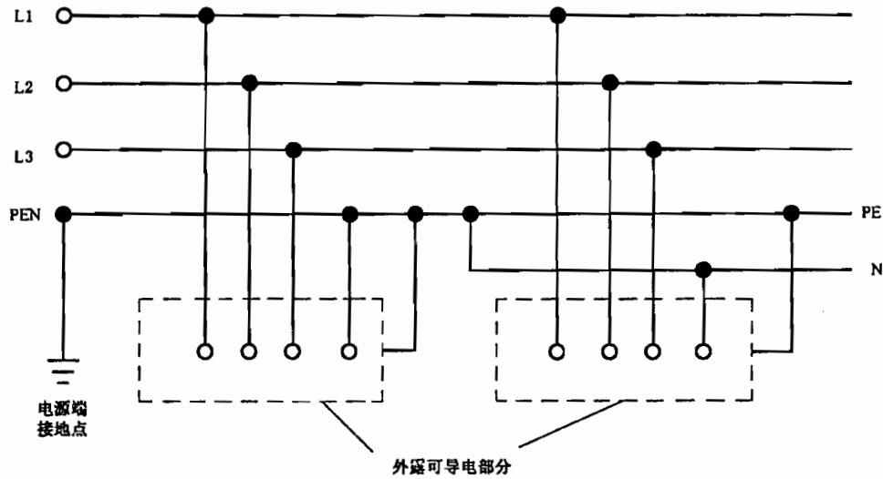
图 3 TN-C-S 系统
