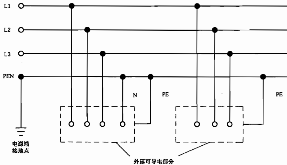
图 2 TN-C 系统
