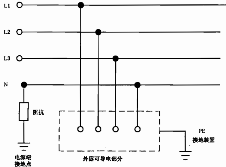
图 5 IT 系统
