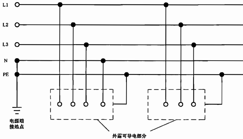
图 1 TN-S 系统
