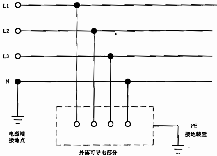
图 4 TT 系统
